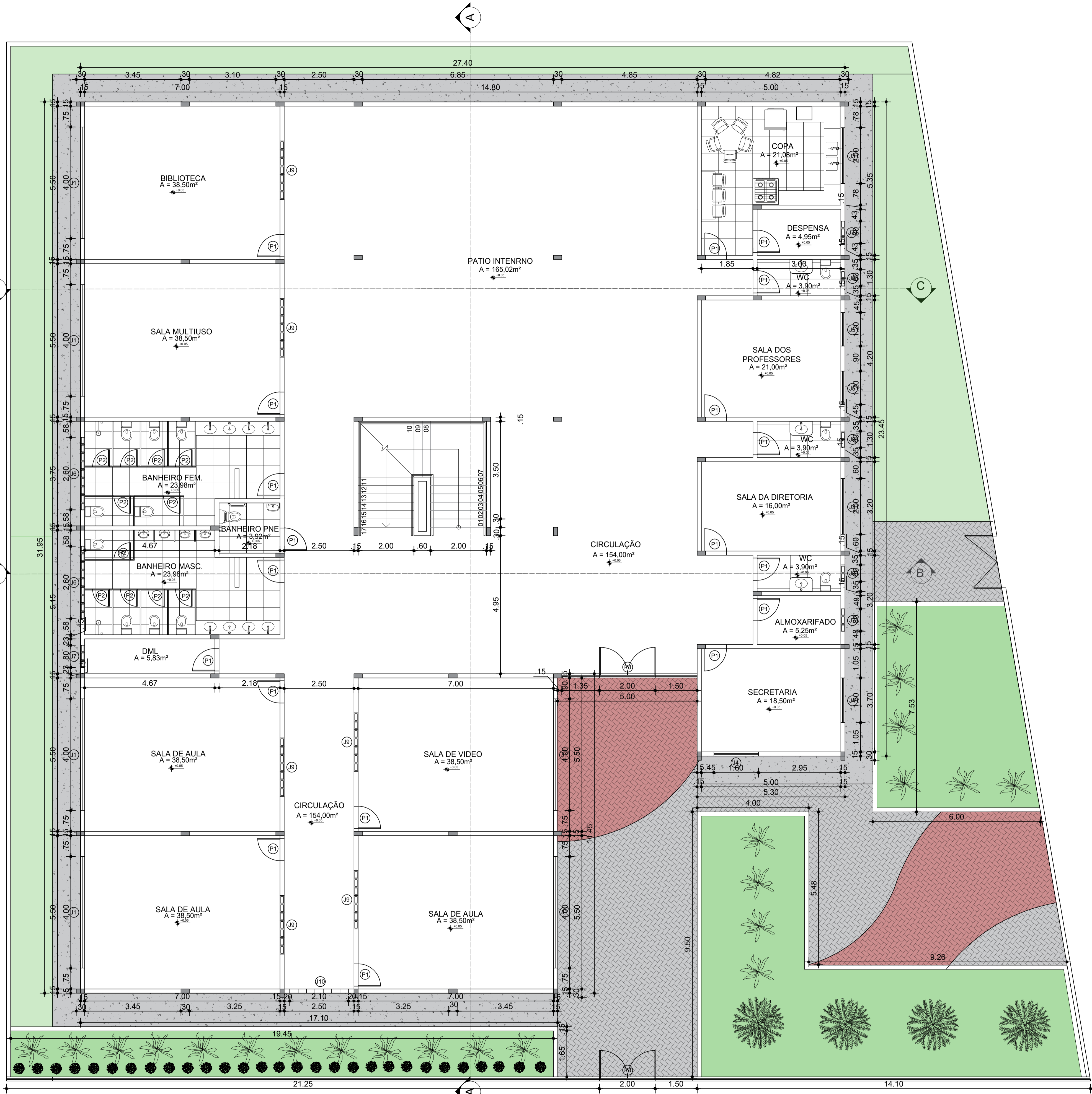
PLANTA BAIXA - PAVIMENTO TÉRREO ESCALA: 1/75
