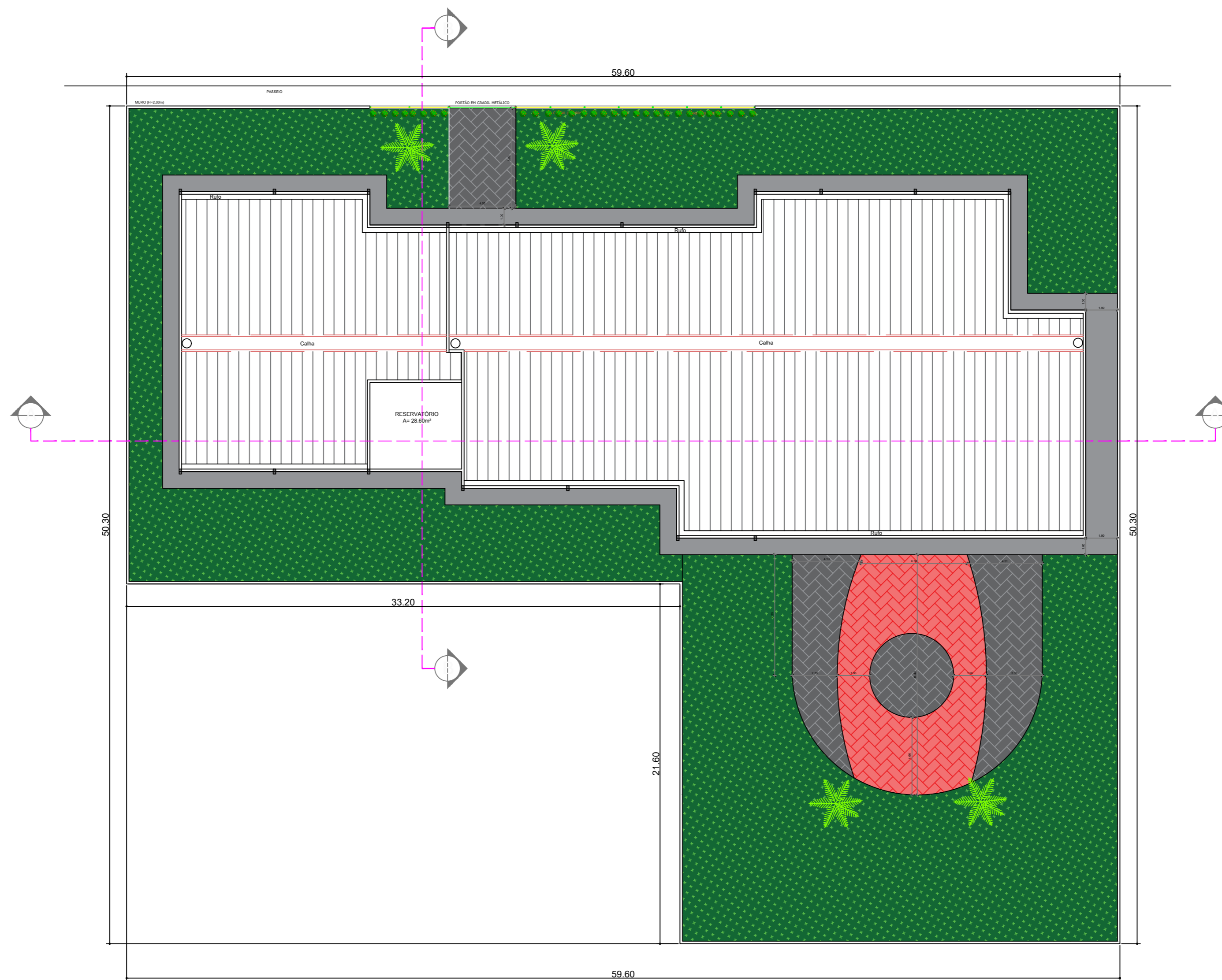
PLANTA DE SITUAÇÃO ESC: 1/200
