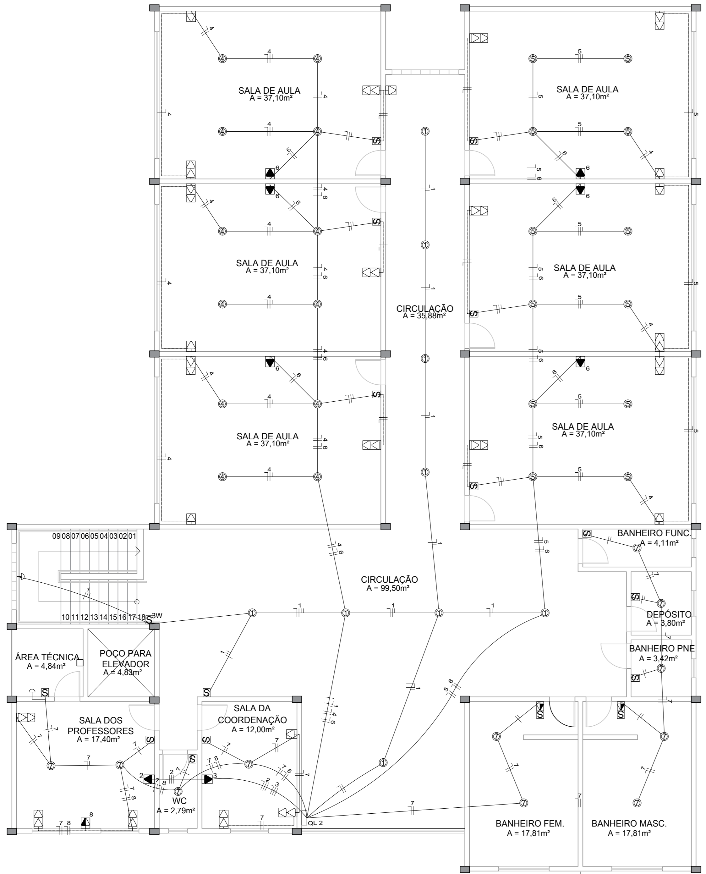
PLANTA DE PROJETO ELÉTRICO - PRIMEIRO PAVIMENTO ESCALA: 1/75
