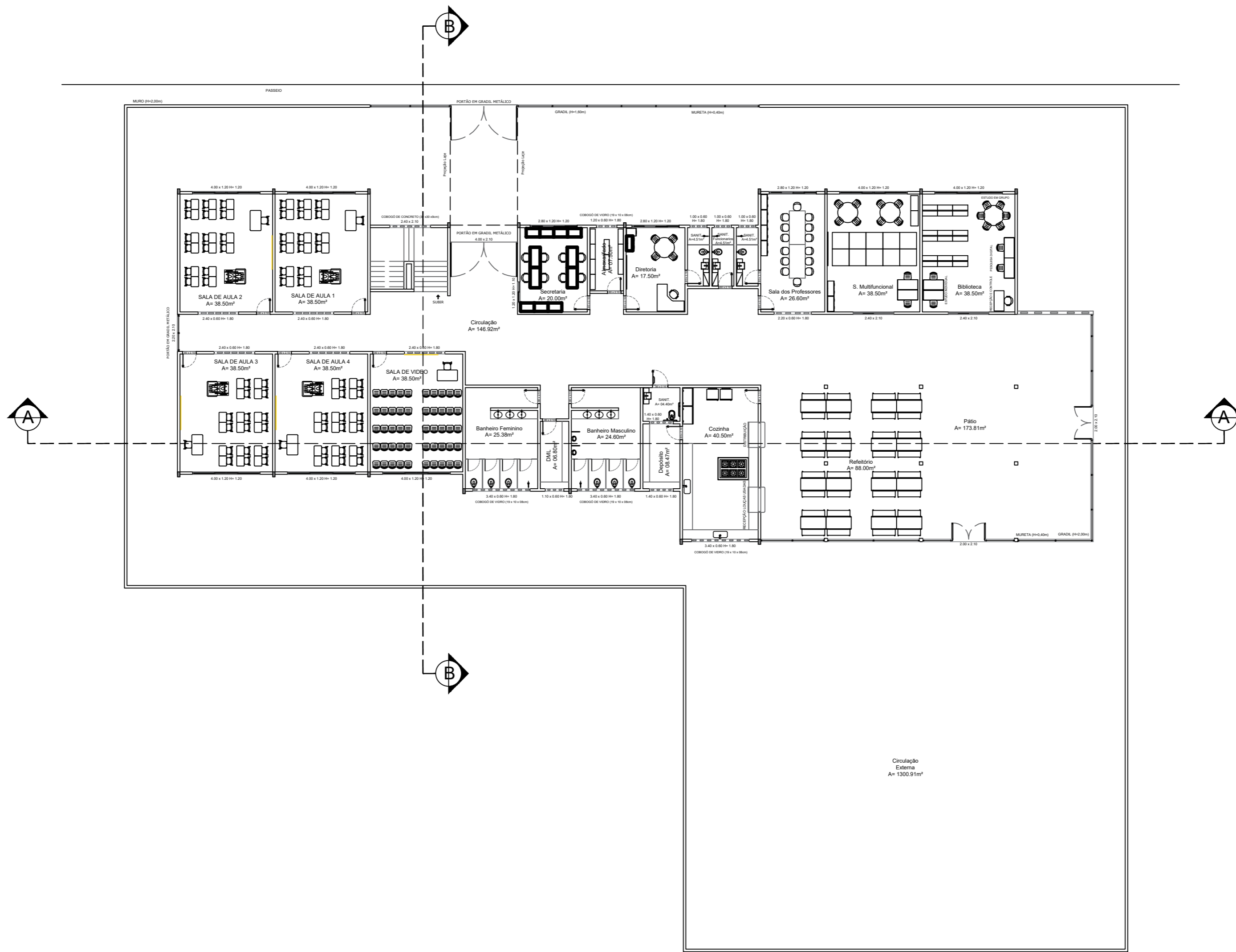
LAYOUT TERREO ESC. 1/200
