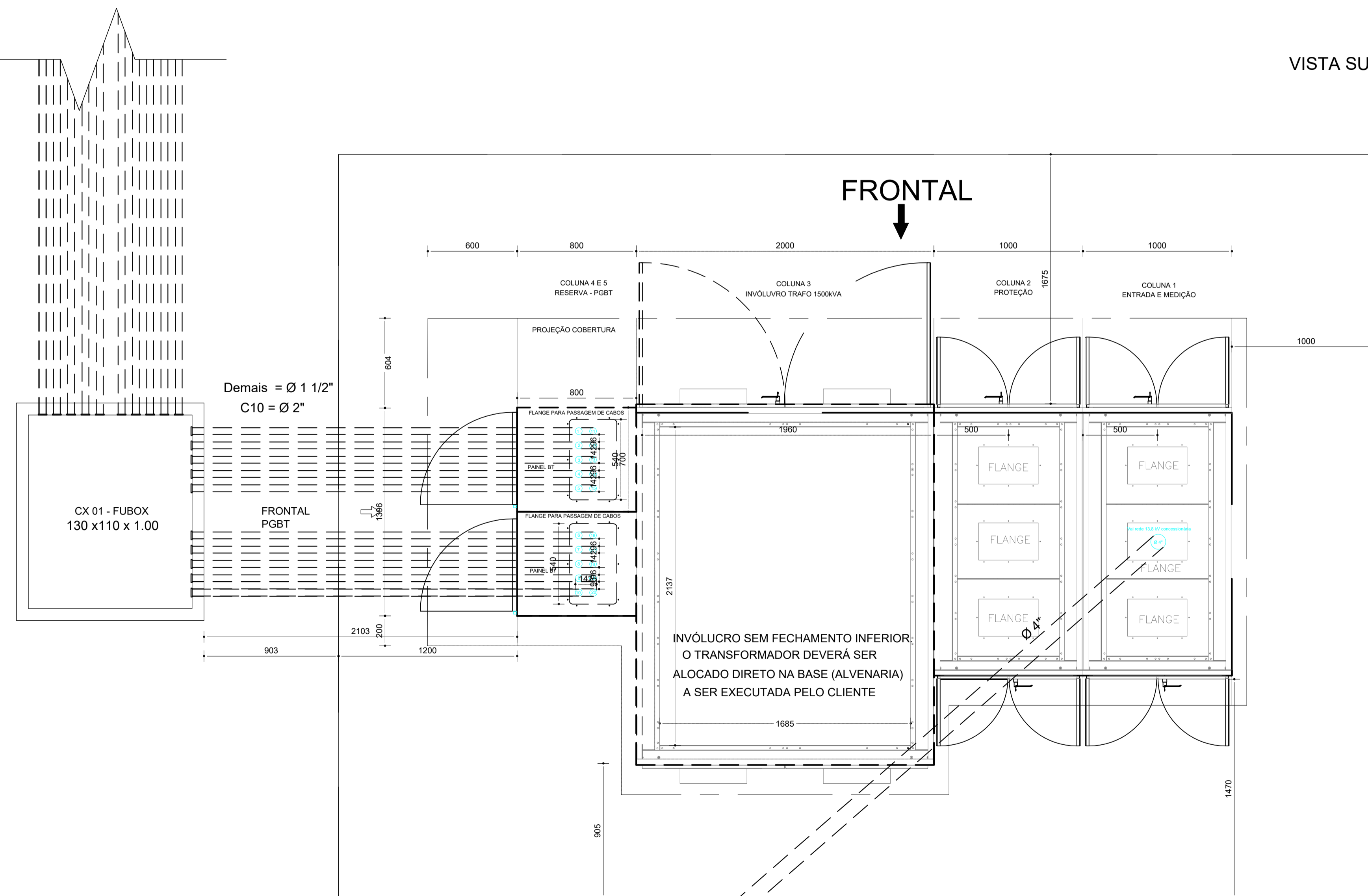
VISTA SUPERIOR INTERNA - DETALHE FLANGE DE ENTRADA / SAÍDA DE CABOS
