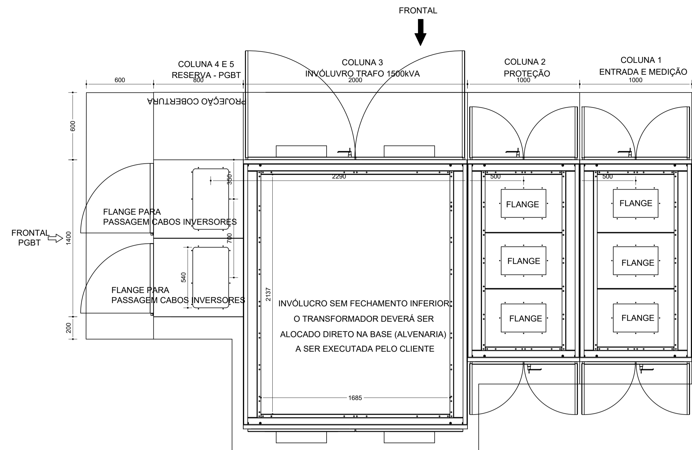
VISTA SUPERIOR INTERNA - DETALHE FLANGE DE ENTRADA / SAÍDA DE CABOS
