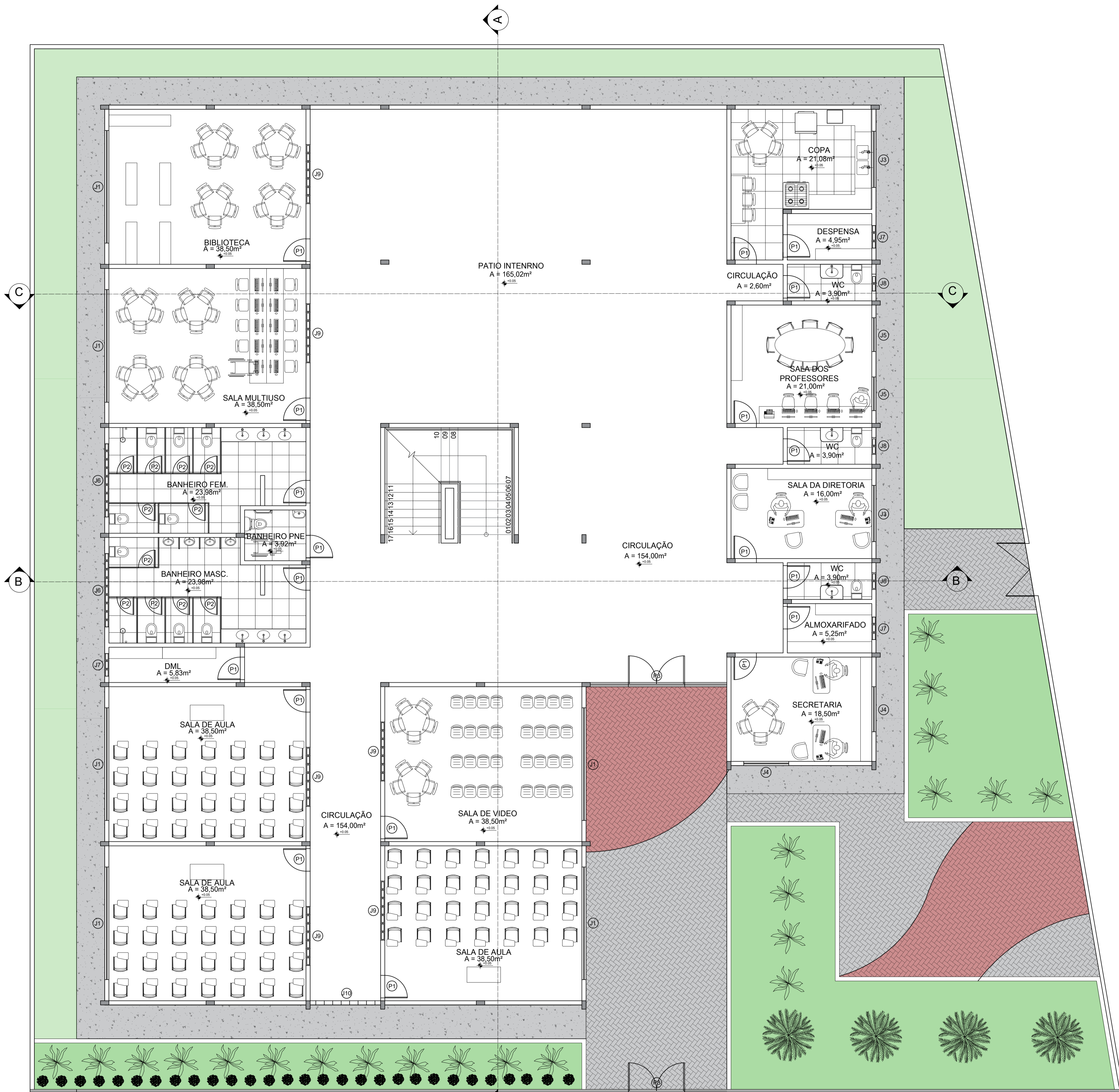
PLANTA DE LAYOUT - PAVIMENTO TÉRREO ESCALA: 1/75
